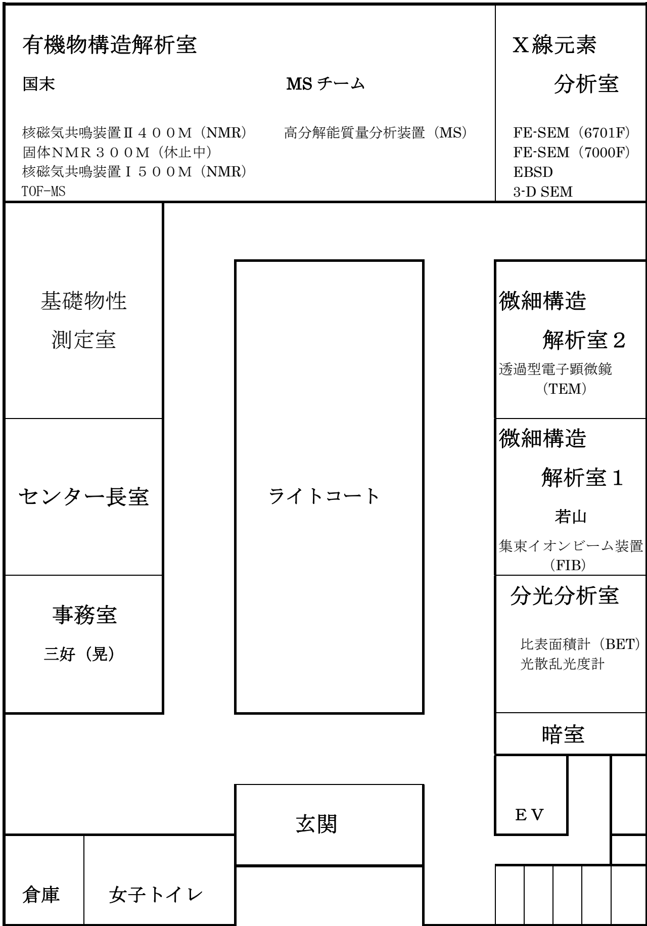
機器分析センター 1階平面図
